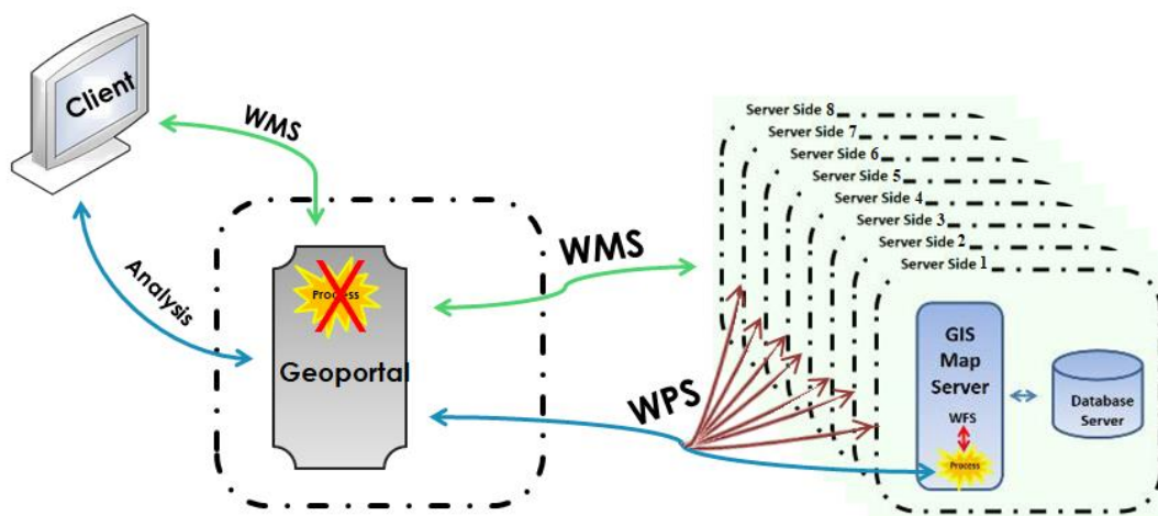
شکل ۳- ساختار پیشنهادی
