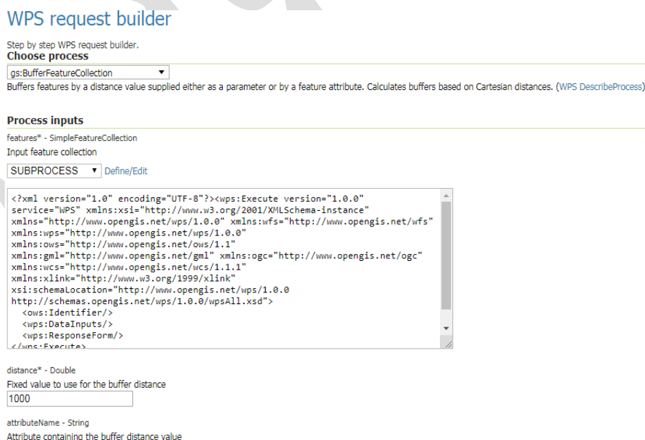
شکل ۷۱- فایل XML حاصل از تحلیل Query به عنوان ورودی تحلیل Buffer
