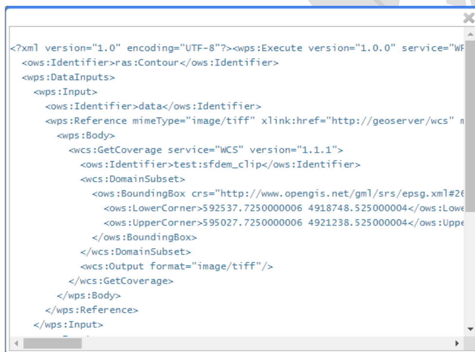
شکل ۶۲- فایل XML حاصل از تحلیل Contains
